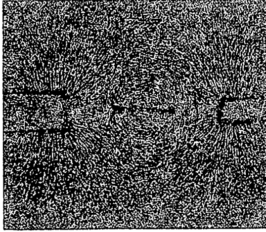
شكل ٢-٩ برادة الحديد تلمع فوق صفحة ورقية مع مغناطيس موضوع أسفله
