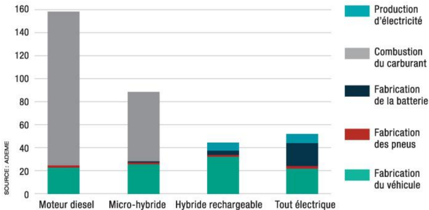
Émissions de CO 2 (en g/km) d'un véhicule léger (catégorie A) en usage urbain en 2030
